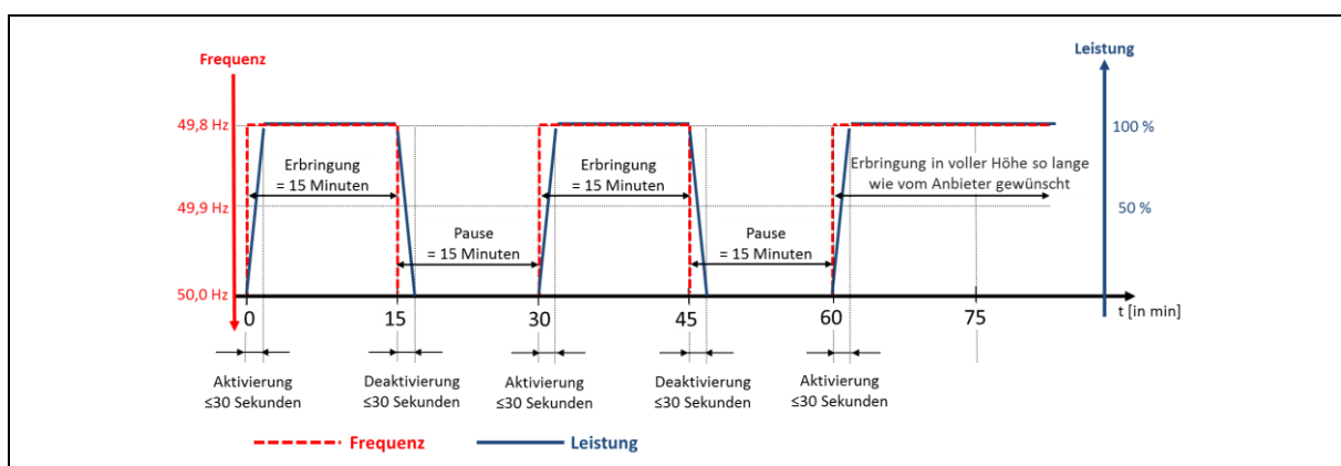
Abbildung 11: Variante 1 des Nachweises des nutzbaren Arbeitsvermögens (FCR)
