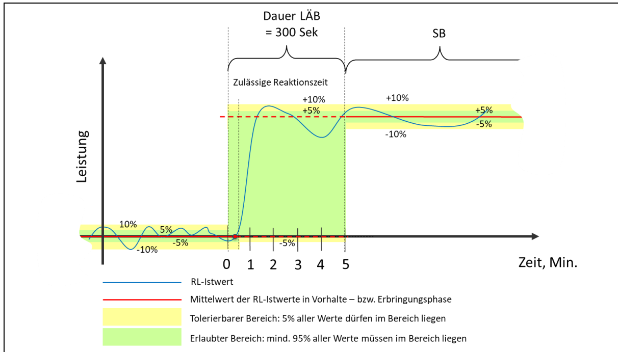
Abbildung 8: Schematische Darstellung der "erlaubten" und "tolerierbaren" Intervalle (aFRR)
