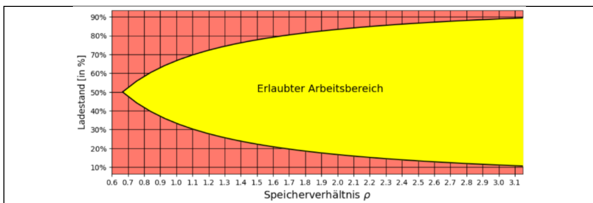
Abbildung 17: Zulässiger Arbeitsbereich bei FCR-E und FCR-G mit begrenzten Energiespeichern
