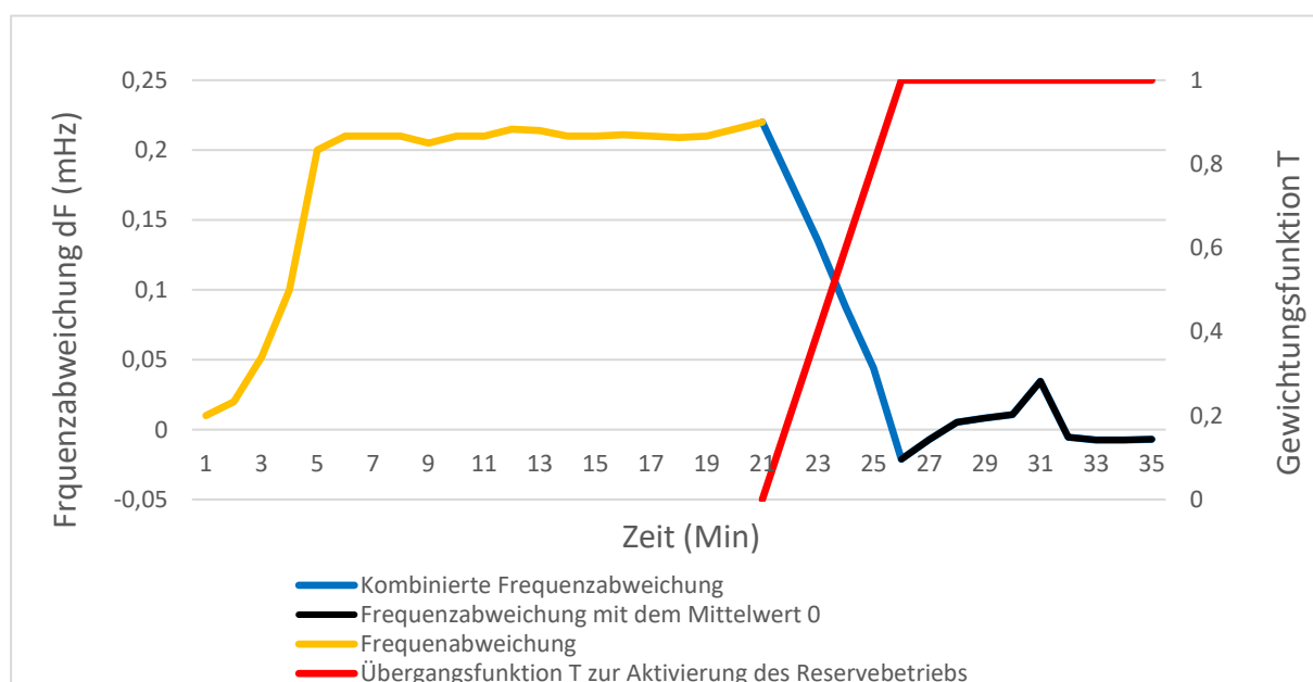
Abbildung 19: Frequenzabweichung im Normal – und Reservebetrieb
